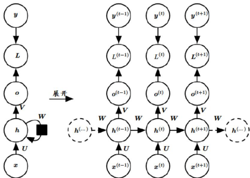
图表1：RNN的展开表示
