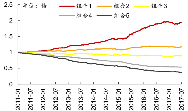
图表28: LSTM 分类模型各层组合净值除以基准组合净值示意图
