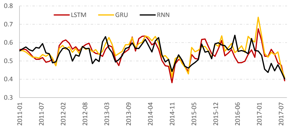
图表17: 三种模型样本外 AUC 变化
