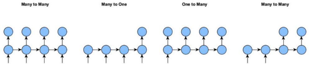
图表2: RNN 的主要形式
